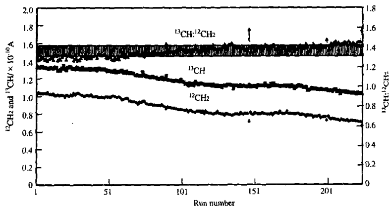
图 1 F- 交替加速时, ^{13}\text{CH} 、 ^{12}\text{CH}_2 束流和 ^{12}\text{CH}_2/^{13}\text{CH} 比值随测量循环次数的变化
